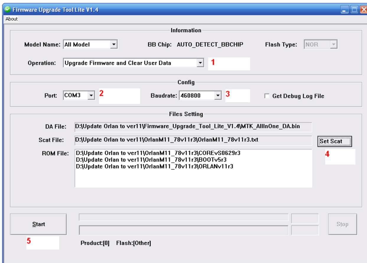
Рис.2 Общий вид программы обновления микропрограммы (прошивки) устройства «Орлан-М11»
